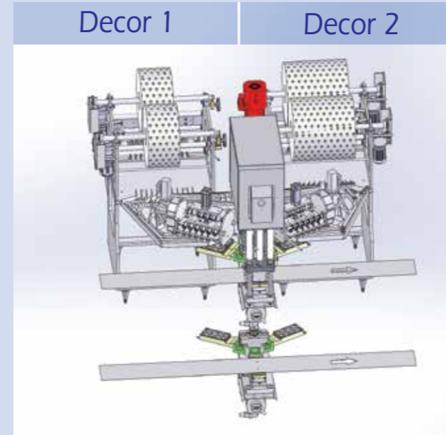
Aplicador de decor Decor labelling
