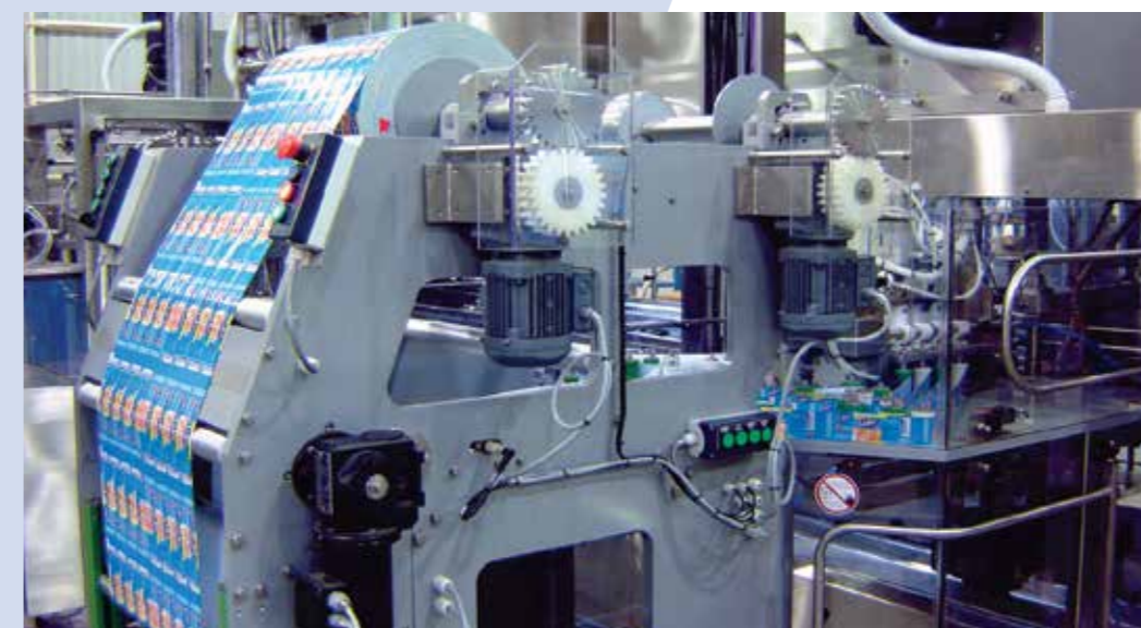
Aplicador de decor Decor labelling
